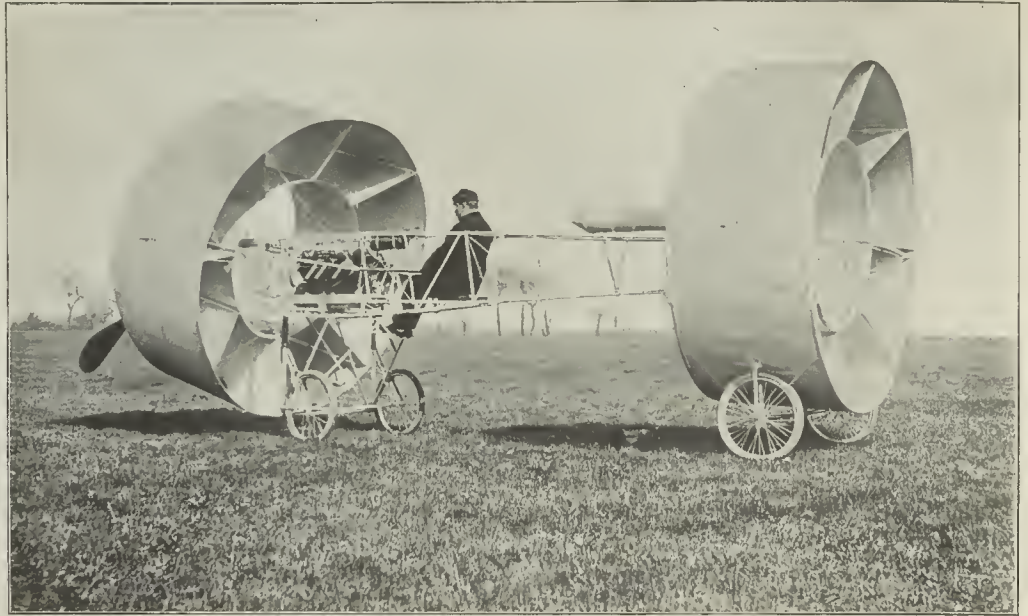
El nuevo aeroplano Givaudán, ensayado recientemente en Villefranche (departamento del Ródano) con éxito satisfactorio (De fotografía de M. Rol y C.º)
